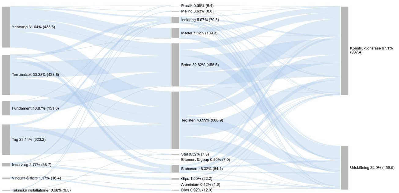
FIGUR 46. Mængder for enfamiliehus 2 for konventionel byggeskik (Enf.02) med en 100-årig betragtningsperiode for produktionsfasen og udskiftninger.
